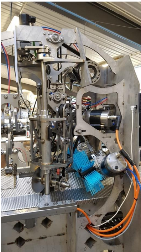
Figur 10. Kutterigg for ørebeinskutt.
